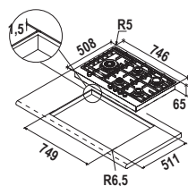
INSTALLAZIONE FILOTOP
